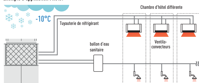
Aucune résistance électrique supplémentaire requise. * Ce dispositif est également valable avec le module hydraulique.
